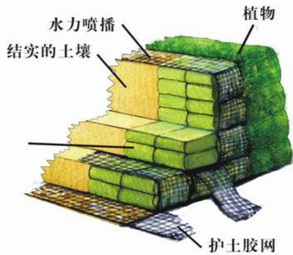
泥质护土墙
