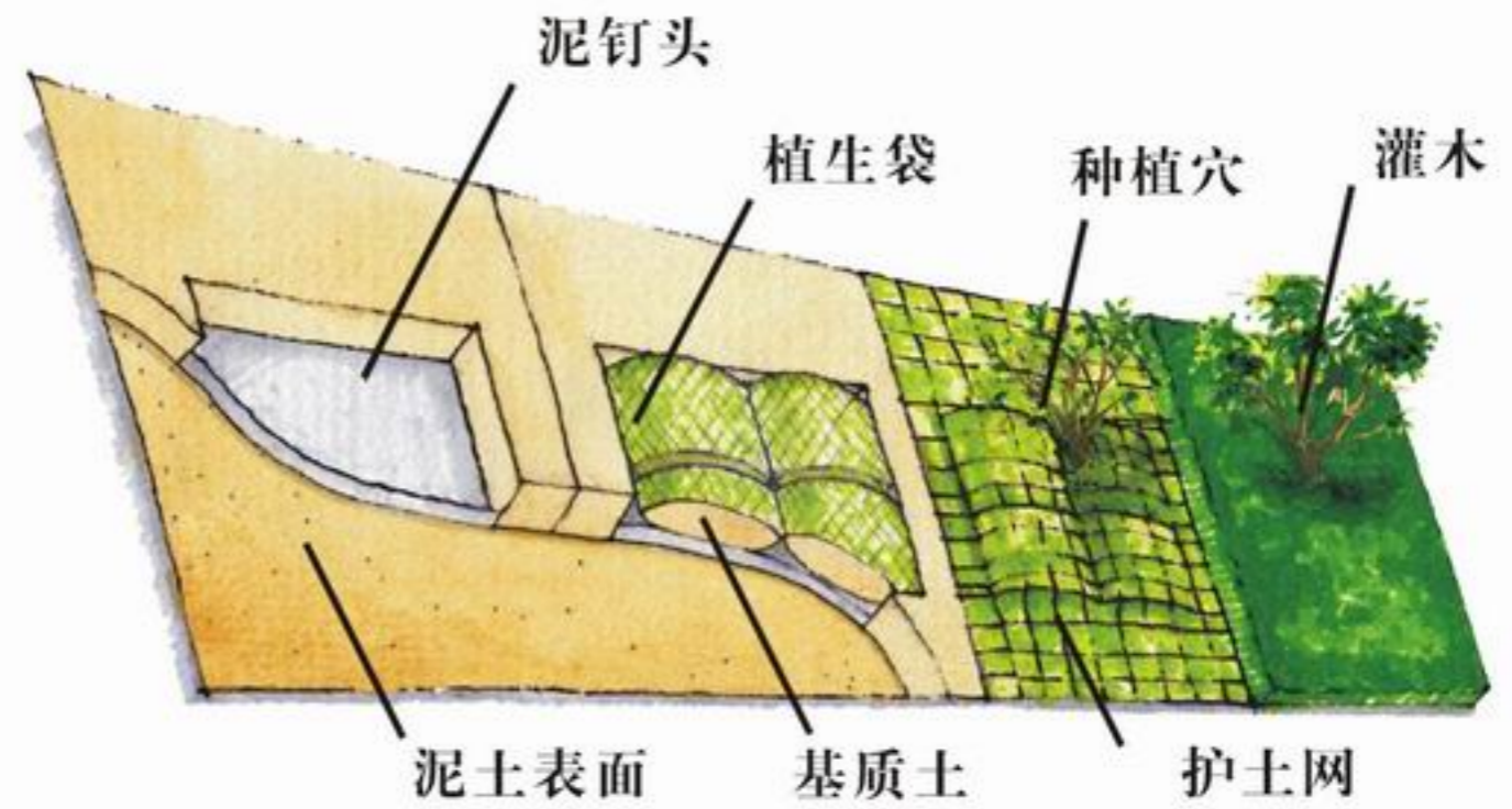
泥钉头
